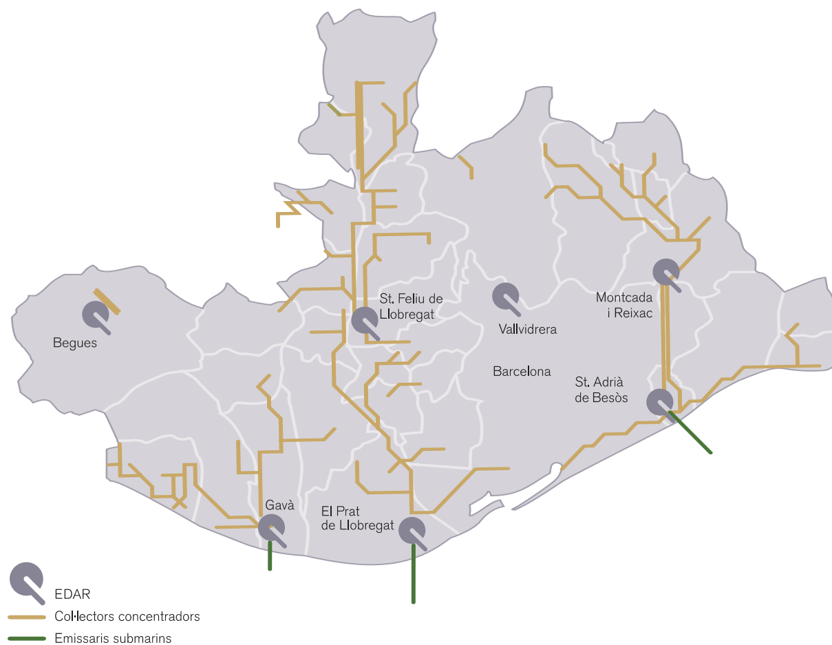
Figura 25 EDAR i principals col·lectors del sistema de sanejament metropolità
